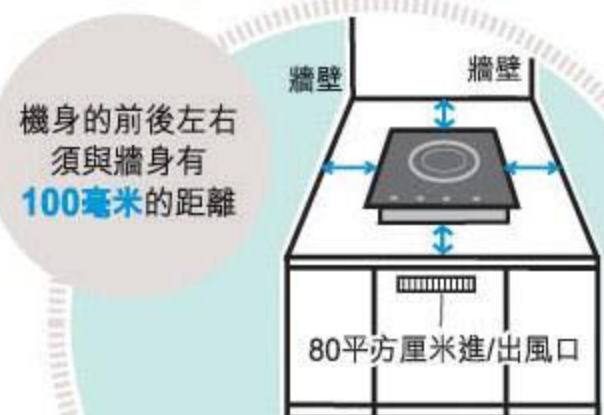
RIC-C26B 安裝圖
